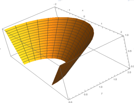
Superficie con dirección principal canónica en \mathbb{R}^3
