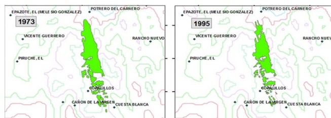
Figura 1: Conceptos fundamentales de la conectividad del paisaje. Un menor hábitat disponible, solo es capaz de mantener poblaciones pequeñas. Caso contrario en las especies de mayor tamaño que requieren hábitats con mayor superficie. Elaboración propia con base en CESAJ y SIGAAF, 2020.
